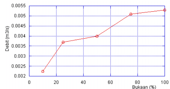
Gambar 4. Pengaruh bukaan katup terhadap kapasitas pompa
