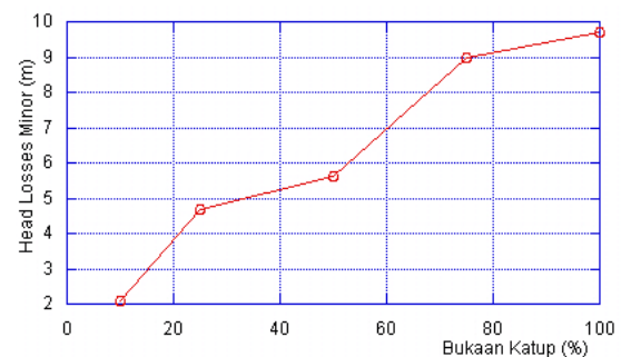
Gambar 7. Grafik pengaruh bukaan katup terhadap head losses minor pada pompa tunggal
