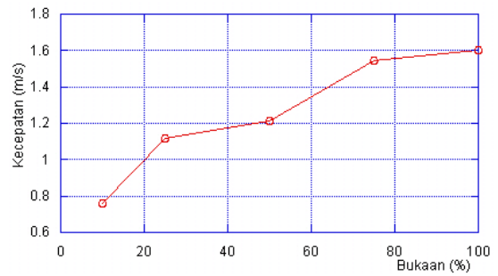
Gambar 5. Grafik pengaruh bukaan katup terhadap kecepatan air pompa tunggal
