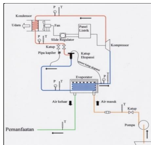
Gambar 5 Skema aliran sistem pendingin water chiller
