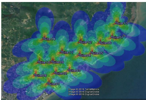
Gambar 11. Coverage area dalam Google Earth
