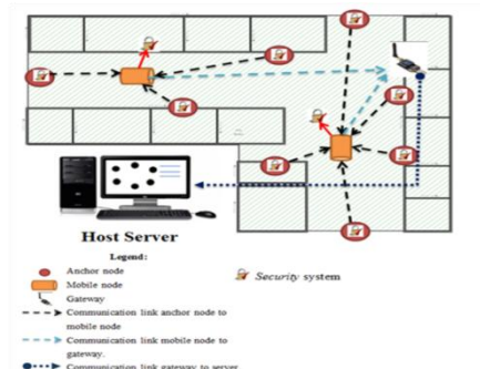
Gambar 1. Skenario Pengujian Secure Indoor Localization System tanpa menggunakan attacker (penyerang)
