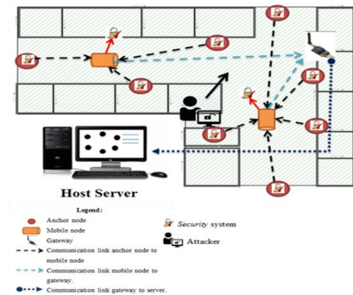
Gambar 2. Skenario pengujian Secure Indoor Localization System dengan menggunakan attacker (penyerang)
