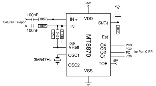
Gambar14 Dekoder DTMF Dan Deteksi Dering
