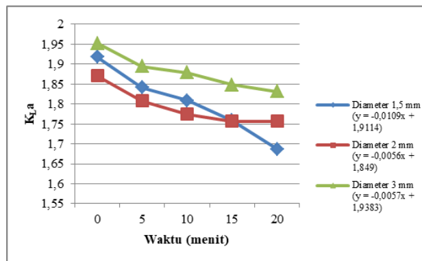
Gambar 3. Grafik K_{La} transfer oksigen.
