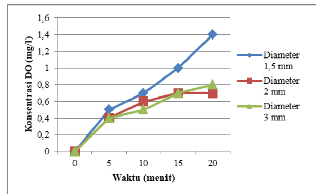
Gambar 2. Grafik hubungan konsentrasi DO dan waktu aerasi pada setiap ukuran diffuser .
