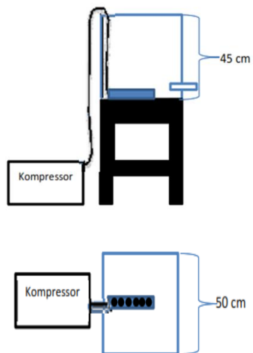
Gambar 1. Skema alat
