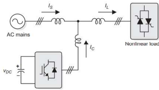
Gambar 5. Topologi SAPF
