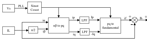
Gambar 7. Blok Diagram Proses Ekstraksi Harmonisa
