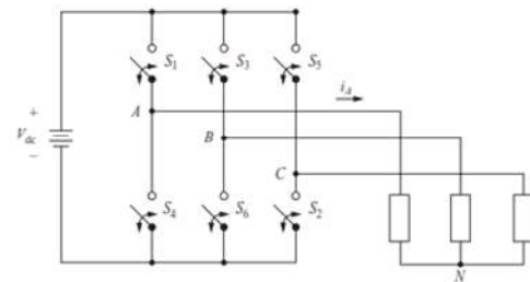
Gambar 3. Rangkaian Inverter Tiga Fasa
