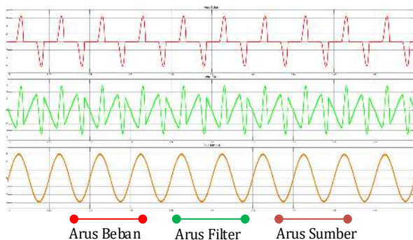
Gambar 12. Gelombang Pengamatan (PI-SAPF Motor 370 W)
