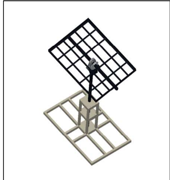
Gambar 5.3D desain keseluruhan
