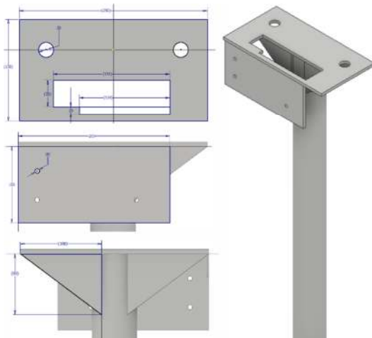
Gambar 8. Desain 3D dudukan komponen sistem transmisi bidang horizontal.
