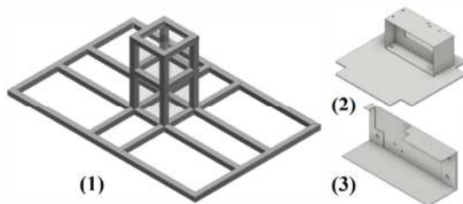
Gambar 9. Desain 3D komponen kaki-kaki.
