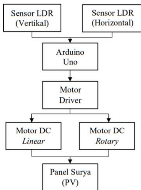
Gambar 2. Diagram blok pengujian.
