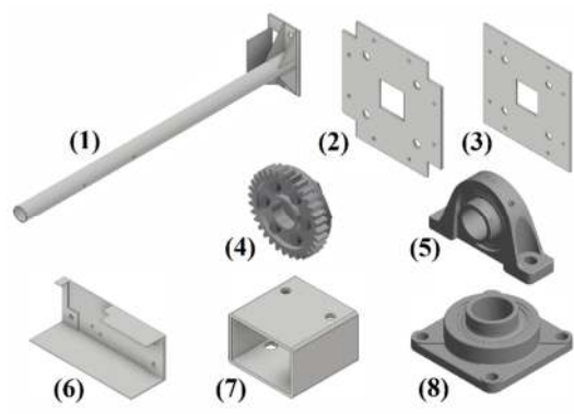
Gambar 7. Desain 3D komponen sistem mekanik bidang vertikal.
