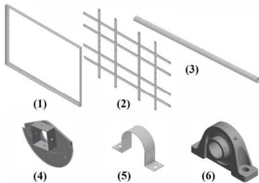
Gambar 6. Desain 3D komponen sistem mekanik bidang horizontal.
