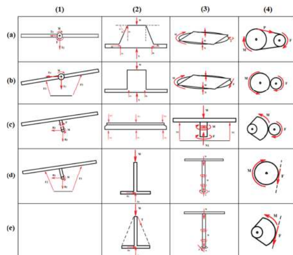
Gambar 3. Skema klasifikasi alternatif desain komponen sun tracker .
