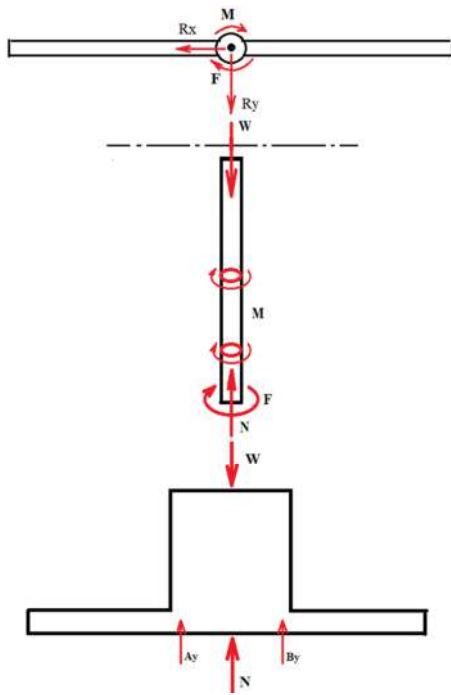
Gambar 4. Free-body diagram desain konsep terpilih.
