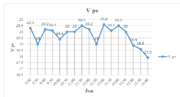
Gambar 5. Grafik Pengujian Tegangan dengan Solar Tracker
