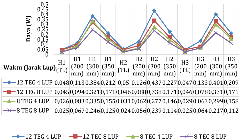
Gambar 4. Grafik Daya Terhadap Waktu dan Jarak Lup
