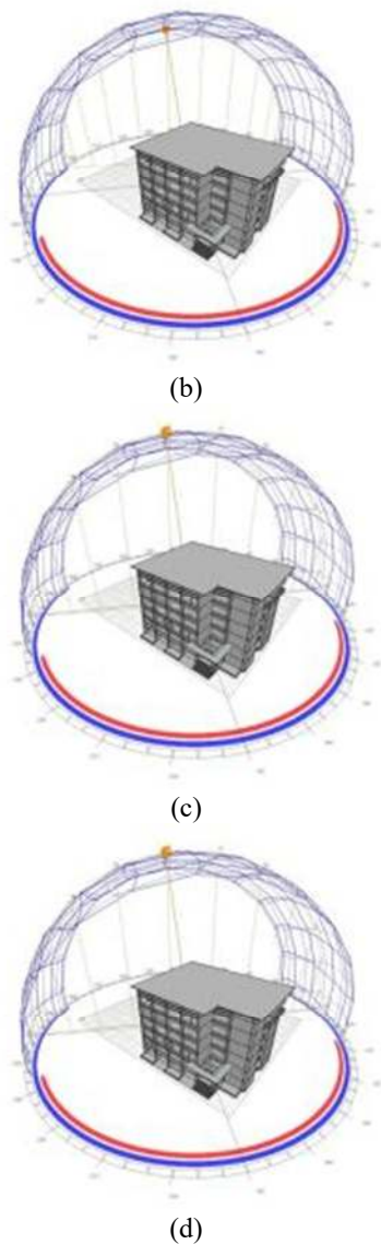
Gambar 5. Permodelan ecotect untuk mendapatkan nilai SC (a) 21 Maret (b) 22 Juni (c) 23 September (d) 22 Desember
