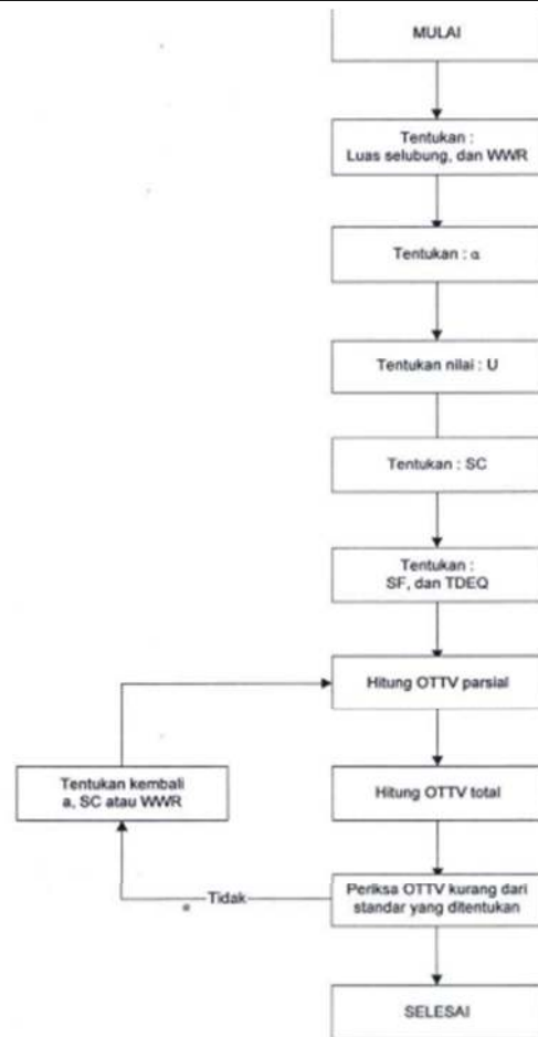
Gambar 4. Bagan kalkulasi OTTV Sumber: SNI 6389:2011
