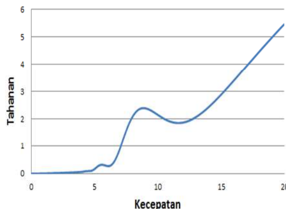
Gambar 3. Perbandingan Tahanan dan Kecepatan Menggunakan Metode Van Ommersen
