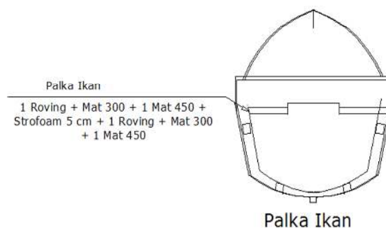
Gambar 11. Detail penggunaan material kapal pada palka
