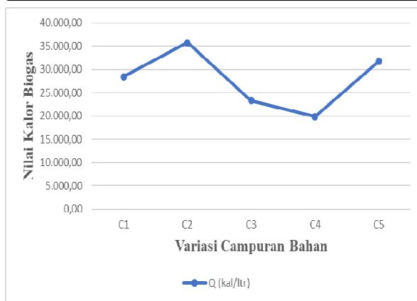
Gambar 5. Grafik nilai kalor biogas
