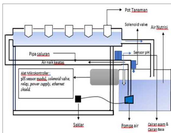
Gambar 3. Desain Alat dan Langkah Kerja
