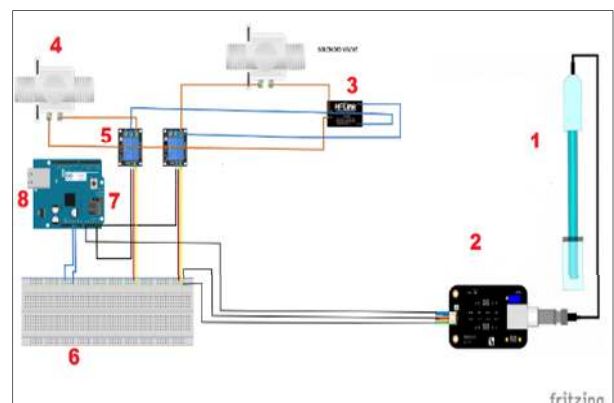
Gambar 4. Desain Perangkat Keras
