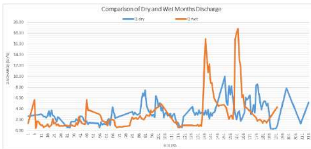
Gambar 6. Hidrograf Debit Observasi Jam-jaman Sungai Bomo untuk Musim Basah dan Musim Kering
