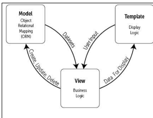
Gambar 2. Arsitektur Model-View-Template
