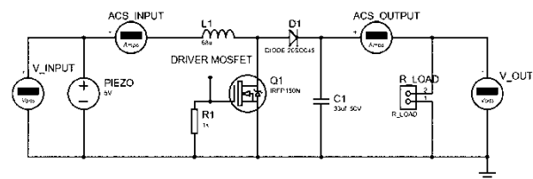
Gambar 5. Rangkaian Boost Converter
