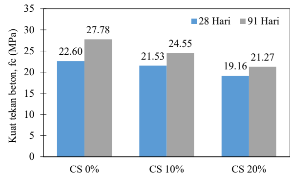
Gambar 6. Kuat tekan beton
