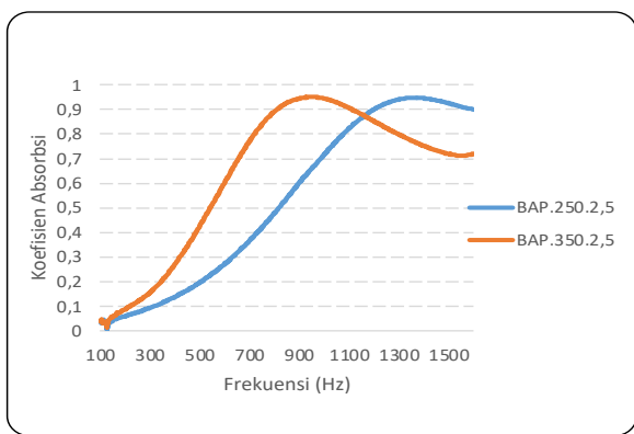
Gambar 2. Kurva perbandingan material dengan perbedaan densitas
