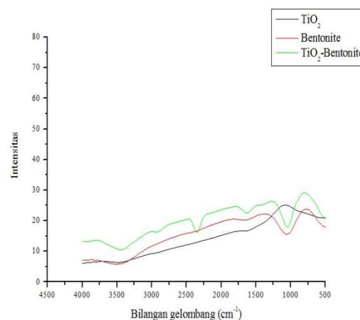
Gambar 2. Spektra FTIR sampel TiO 2 , bentonit, dan TiO 2 -bentonit
