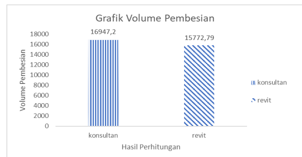
Gambar 1. Grafik Perbandingan Volume Pembesian
