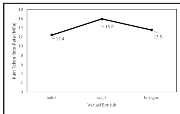
Gambar 2. Grafik pengujian Kuat Tekan Rata-rata komposisi 30:70
