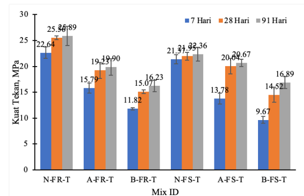
Gambar 2. Kuat tekan mortar pada umur 7, 28, dan 91 hari
