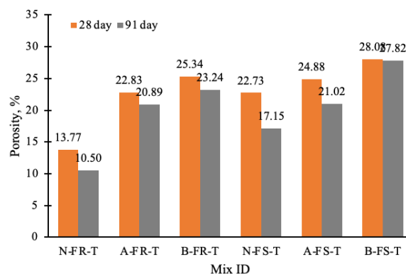
Gambar 3. Porositas mortar pada umur 28 dan 91 hari
