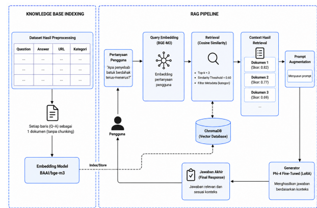
Gambar 2. Arsitektur RAG
