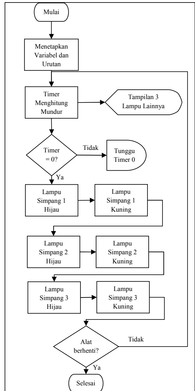
Gambar 1. Diagram Alir Kerja Alat
