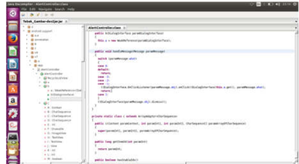
Gambar 9. Source code hasil dekompile menggunakan aplikasi JD-GUI
