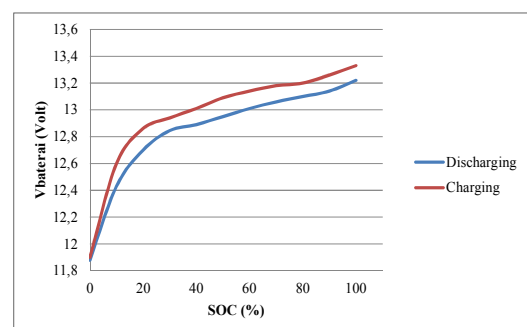
Gambar 8. Kurva karakteristik OCV-SOC kondisi charge-discharge
