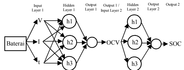
Gambar 5. Arsitektur pemodelan FF-BPNN sebagai estimasi SOC baterai
