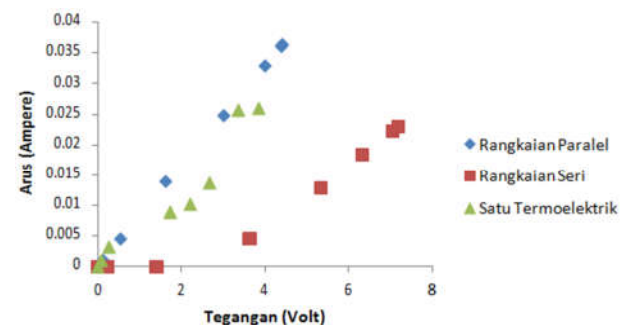
Gambar 4. Hubungan Nilai Tegangan dan Nilai Arus
