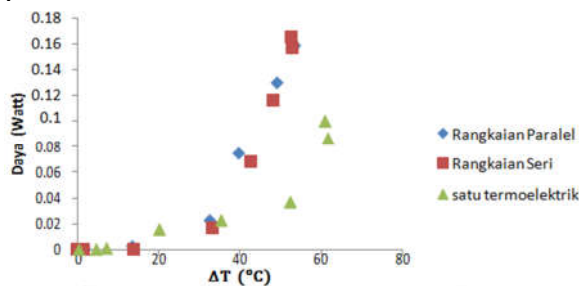
Gambar 5. Hubungan Perbedaan Suhu dengan Nilai Daya
