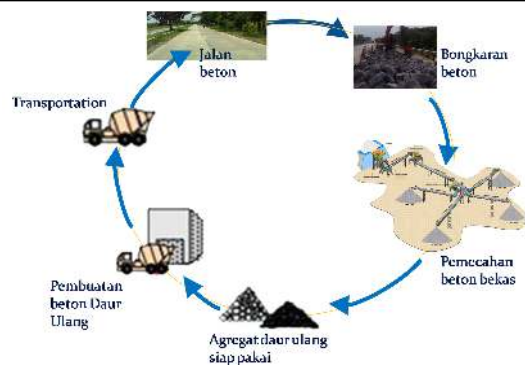
Gambar 2. Proses pembuatan agregat daur ulang dari bongkaran perkerasan kaku jalan raya
