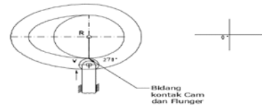
Gambar 12. Posisi Cam menjelang naik dengan sudut 270°
