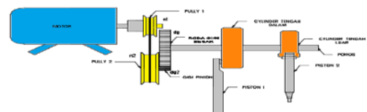
Gambar 2. Skema Alat Mesin Pencetak Tablet
