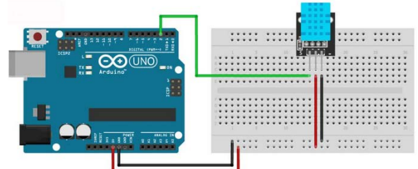
Gambar 5. Pemasangan Sensor DHT11 dengan arduino
