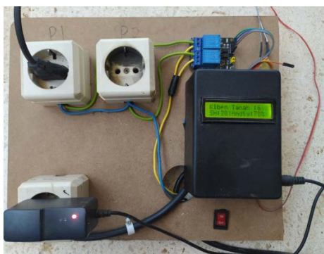
Gambar 10. Kontrol alat
