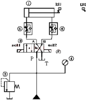
Gambar 3. Diagram Rangkaian Sistem Hidrolik
