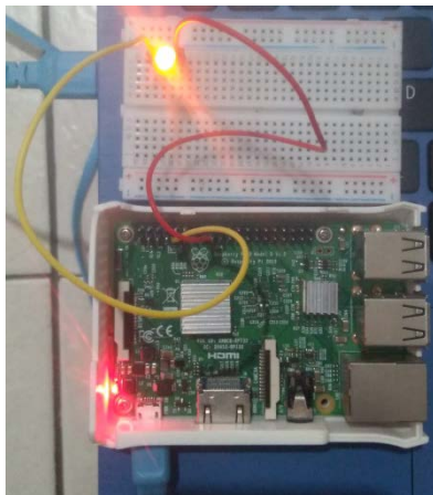
Gambar 6. Pengujian Raspberry Pi
