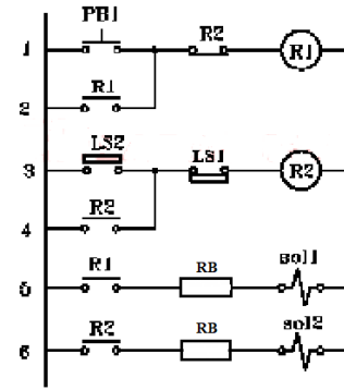
Gambar 4. Diagram Rangkaian Sistem Elektrik
