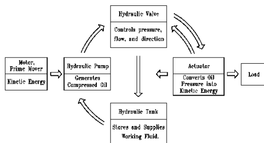
Gambar 1. Diagram Sistem Hidrolik
