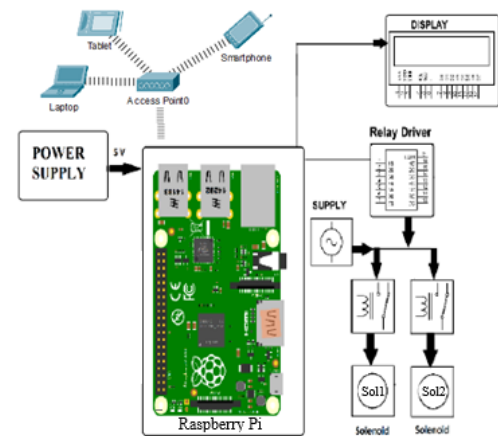
Gambar 5. Diagram Blok Sistem Kontrol dan Monitoring
