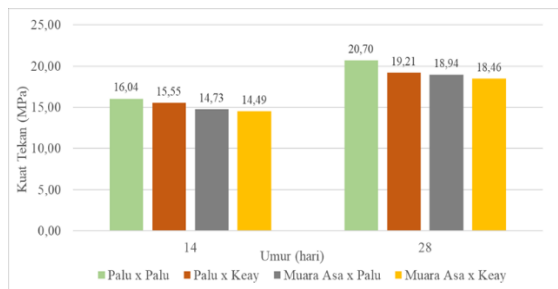
Gambar 2. Grafik Hasil Pengujian Kuat Tekan Beton
