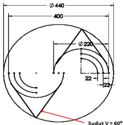
Gambar 2. Geometri turbin angin Savonius dengan variasi kombinasi sudu
