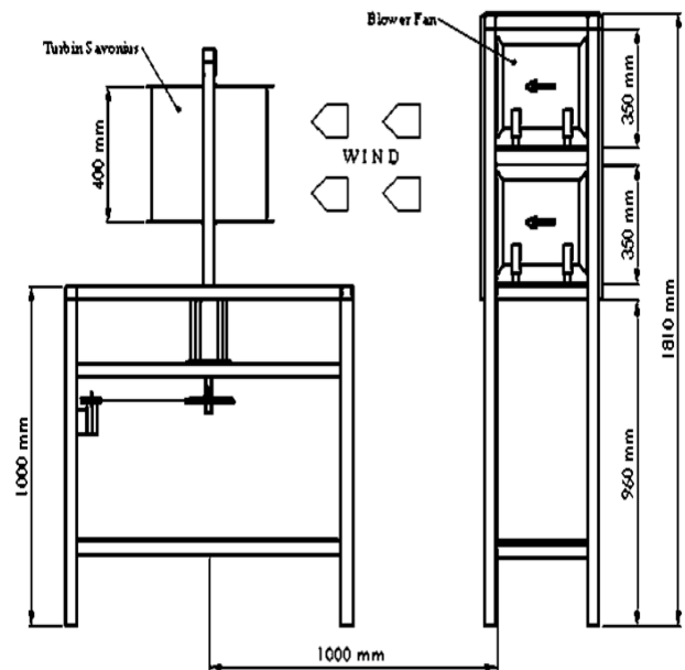
Gambar 3. Skematik pengujian
