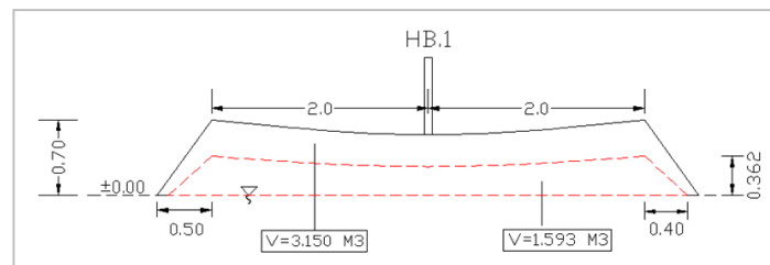
Gambar 10. Ilustrasi Perubahan Volume Tanah pada Sampel HB.1
