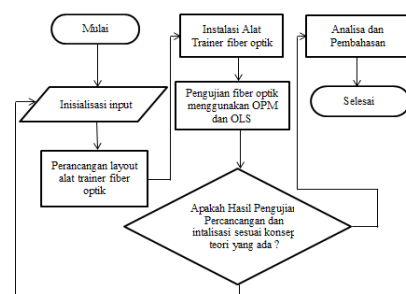
Gambar 2. Flowchart Pengerjaan
