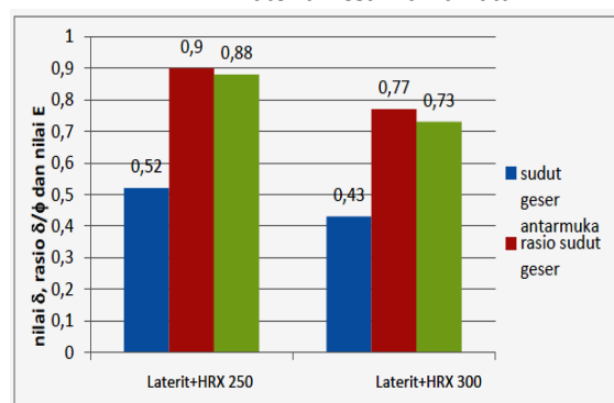
Gambar 8. Nilai Parameter Kekutan Geser Berdasarkan Variasi Penggunaan Geotekstil Tanah Laterit Desa Parigi
