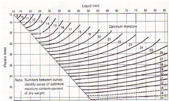
Gambar 1. Grafik untuk perkiraan OMC yang digunakan pada uji kepadatan Proctor standar (Bowles, 1982)
