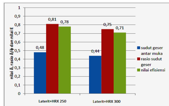
Gambar 7. Nilai Parameter Kekutan Geser Berdasarkan Variasi Penggunaan Geotekstil Tanah Laterit Desa Bukit Batu
