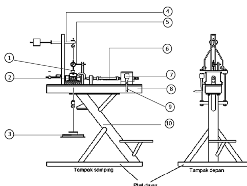
Gambar 2. Alat Uji Geser Langsung (manual)
