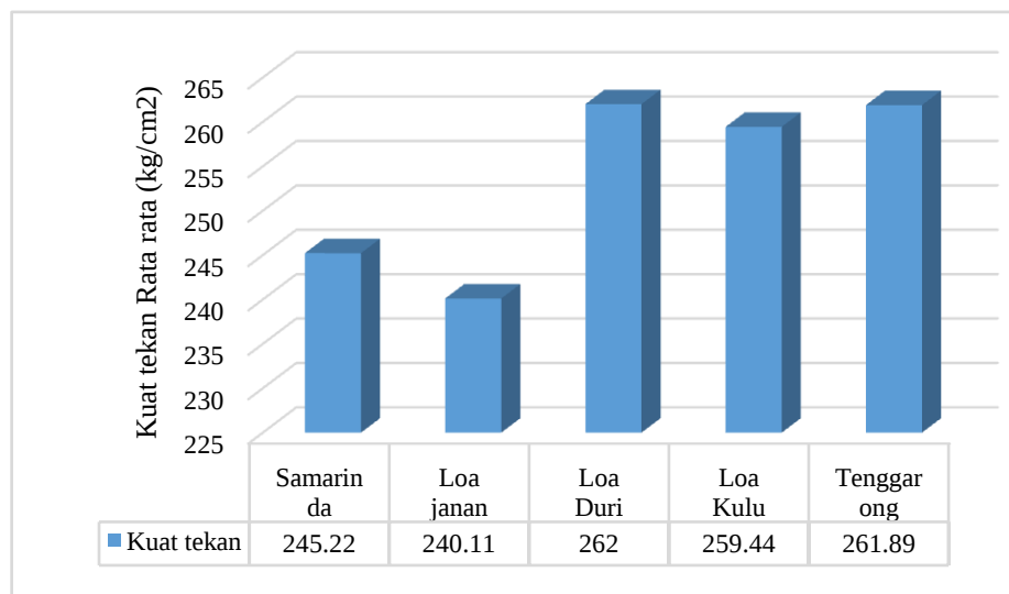
Gambar2. Hasil pengujian kuat tekan rata rata
