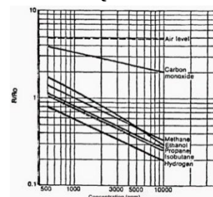
Gambar 2.2 Karakteristik Sensitivitas Sensor MQ-136
