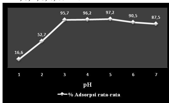
Gambar 3. Kurva pengaruh variasi pH terhadap % adsorpsi Fe.
