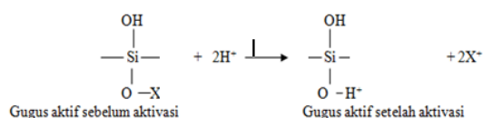
Gambar 1. Proses aktivasi pada abu layang.
