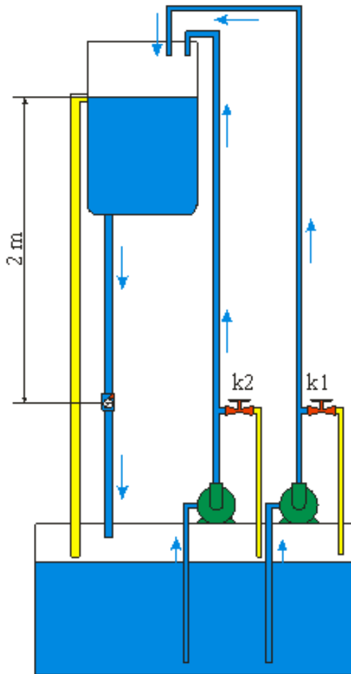
Gambar 3. Skematik Alat
