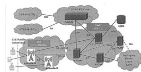
Gambar 2. Arsitektur 4G LTE
