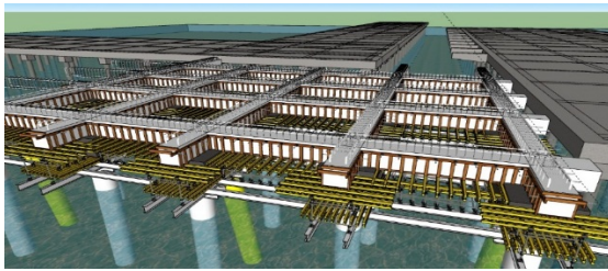
Gambar 9. Ilustrasi Pemasangan Support Bekisting
