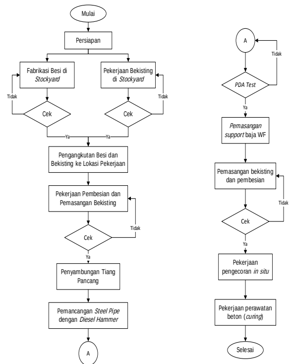
Gambar 6. Diagram alir metode kerja pekerjaan struktur in situ
