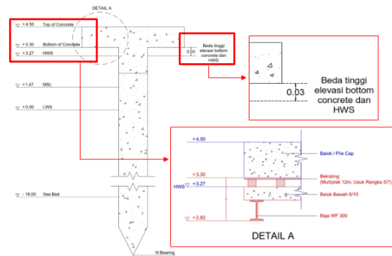
Gambar 10. Profil Elevasi Eksisting (LWS-HWS)
