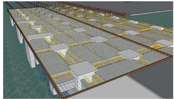
Gambar 17. Ilustrasi Pemasangan Besi In Situ dan Bekisting Stop Cor
