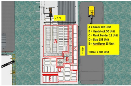
Gambar 13. Layout Penempatan Precast
