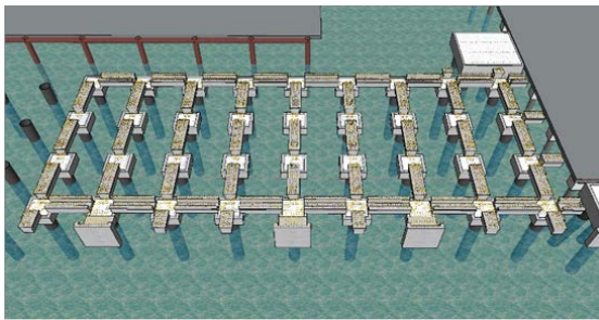
Gambar 15. Ilustrasi pemasangan precast balok melintang
