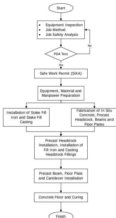
Gambar 14. Diagram alir metode pekerjaan struktur atas Precast
