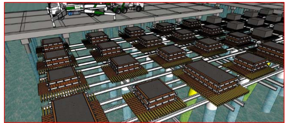
Gambar 8. Ilustrasi Pengecoran Pier / Pile Cap Tahap Kedua
